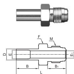
HMFS TBW Body
