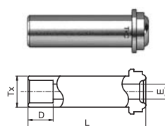
Socket Weld Long Gland
