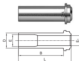
HMFS Long Gland
